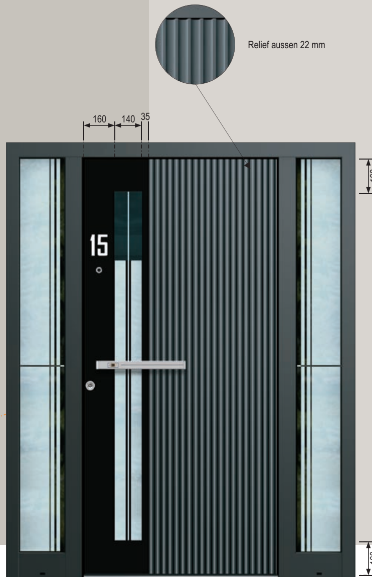
AAE 1590 Dekor bündig nur aussen Relief beidseitig Zubehör Glasmotiv MS 5859 Griff aussen ZAE 141 R Farbe RAL 7012 matt Dekor aussen RAL 9011 FS Hausnummer HE Türspion BT 19 E Seitenteil ST 01 / WG / 400 Glasmotiv MS 5859/S Option: Profilkonstruktion AT 70 Dekor auch innen
