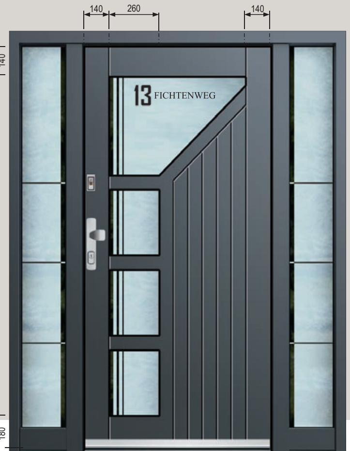
AGE 1822 Relief beidseitig Zubehör Glasmotiv MS 5794 + Hausnummer HFG Griff aussen GA 190 S P Wetterschenkel E-200 Farbe 70 784 FS Seitenteil ST 01 / WG / 400 Glasmotiv MS 5794/S Option Fingerscan
