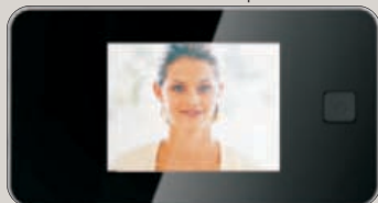
BT 19 E - Elektronischer Türspion - Inneneinheit
