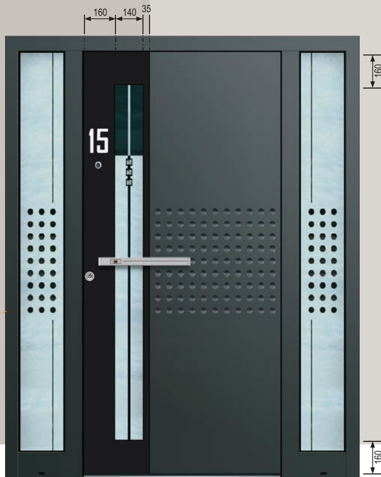
AAE 1582 Dekor bündig nur aussen Relief beidseitig Zubehör Glasmotiv MS 5813 SK - Swarovski Kristall Griff aussen ZAE 141 R Farbe RAL 7012 matt Dekor aussen RAL 9011 FS Türspion BT 19 E Hausnummer HE Seitenteil ST 01 / WG / 400 Glasmotiv MS 5813/S Option: Profilkonstruktion AT 70 Dekor auch innen
